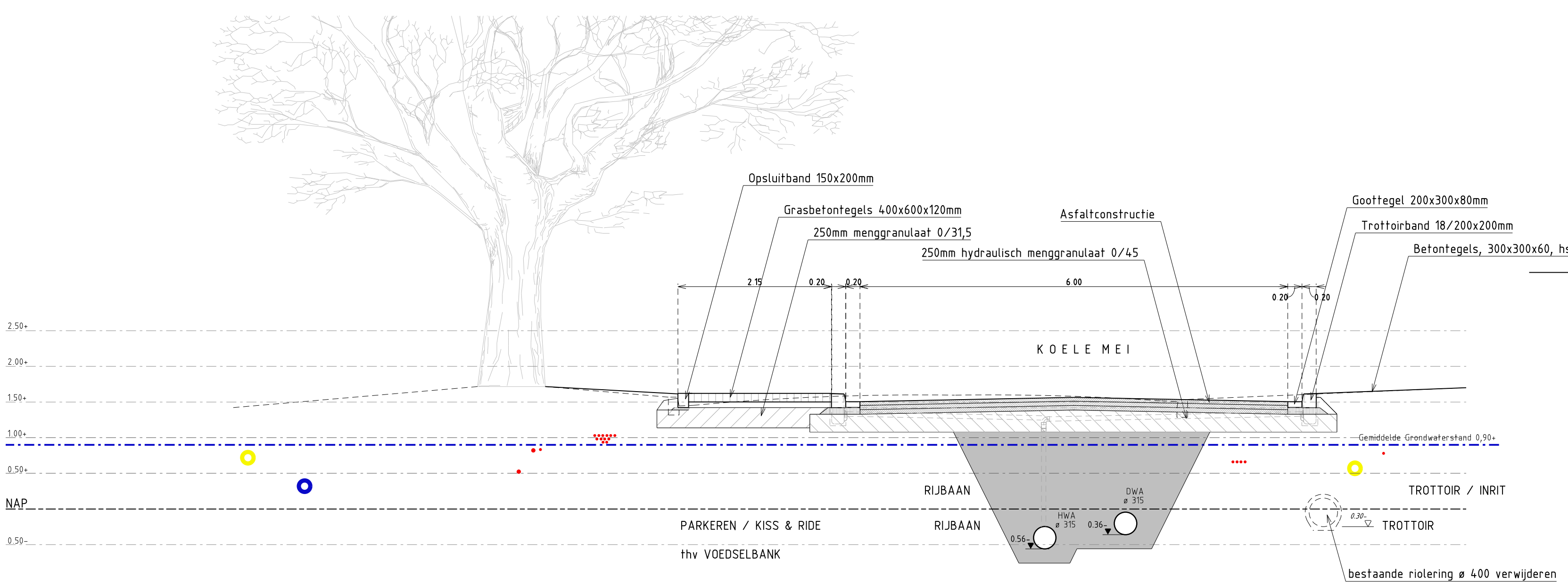
PRINCIPE DWARSPROFIEL 02 KOELE MEI thv hsnr 9
